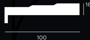
Наличник Ступенчатый 16*100 мм
