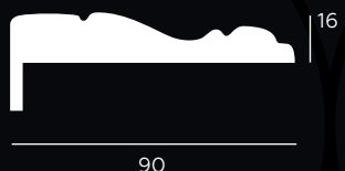
Наличник Фигурный Телескопический 16*90 мм
